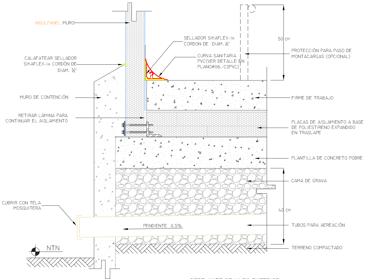
DESPLANTE DE MURO EXTERIOR EN CONGELADOR
