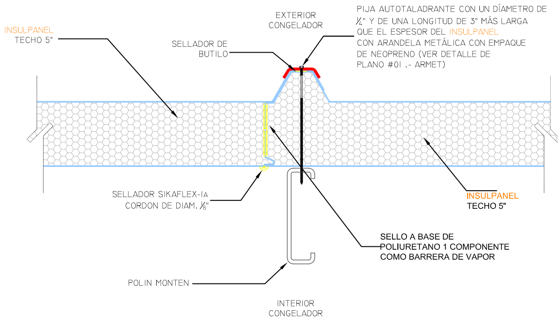
CORTE TRANSVERSAL CUBIERTA CONGELADOR
